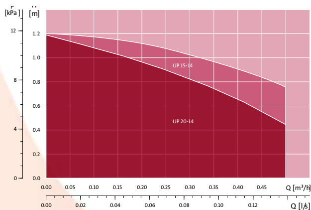
Curvas características de la gama COMFORT.
